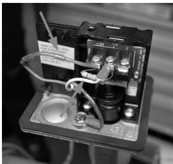
Рис. 3 Пример установки сопротивлений (резисторов) в корпусе реле давления
