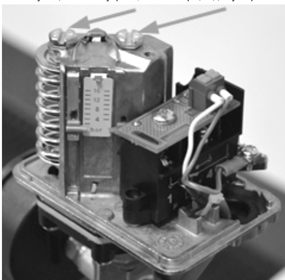
5-сур. FRG-2 қысым релесін баптау
