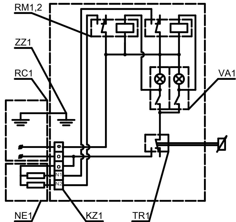
Рисунок 2 Схема ПУЭ-6/02
